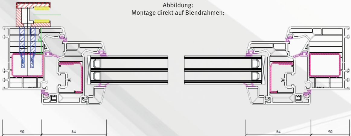
Abbildung: Montage auf Neubau-Rollladenführung (108.158)
